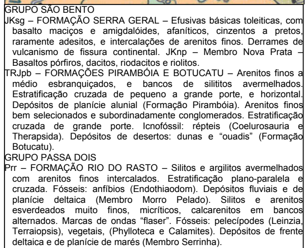
Figura 02 – Mapa geológico da área da Caverna da Homenagem. Fonte MINEROPAR (2001) modificado.
